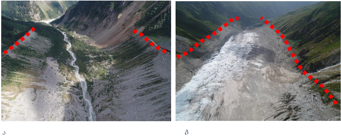
ფიგურა 33. მცირე გამყინვარების პერიოდის მორენული მწკრივები ა) ჭალაათი; ბ) ადიში
